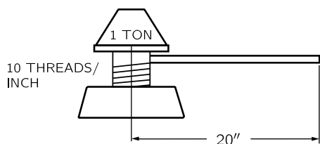
图 4.5: 螺旋起重器
