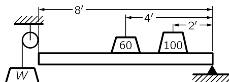
图 4.6: 一端支撑着的荷重杆
