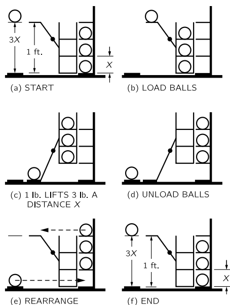
图 4.2: 一种可逆机
