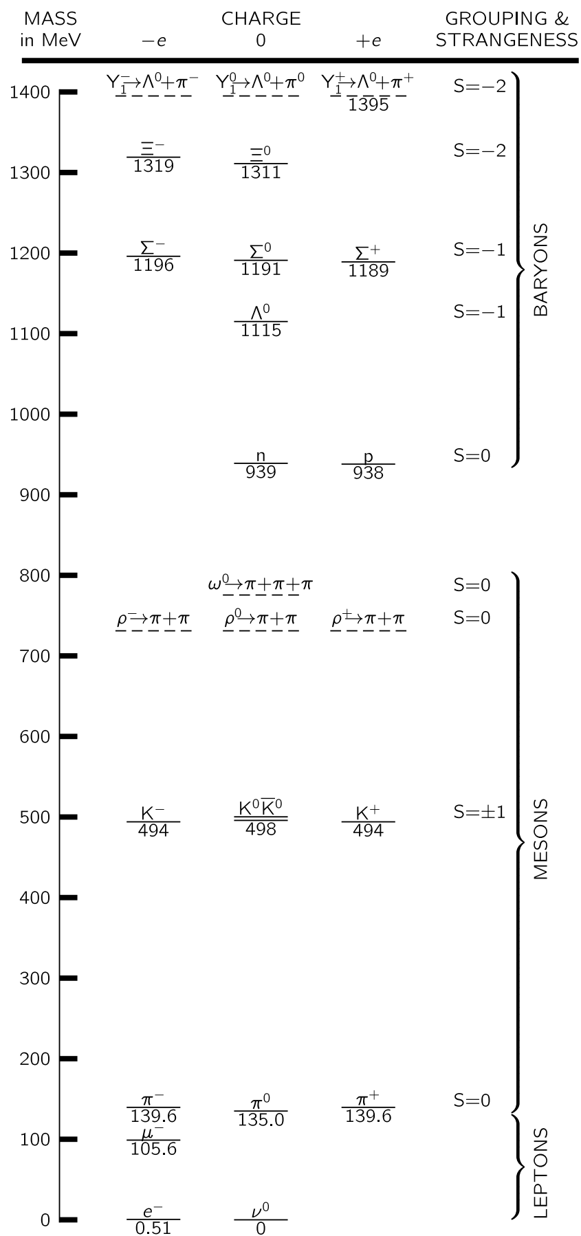
图 2.1: 基本粒子
