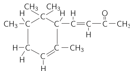
图 1.10: \alpha 鸢尾酮香料的分子结构图
