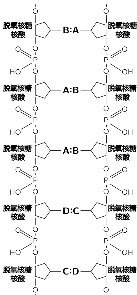
图 3.2: 部分 DNA 分子结构图
